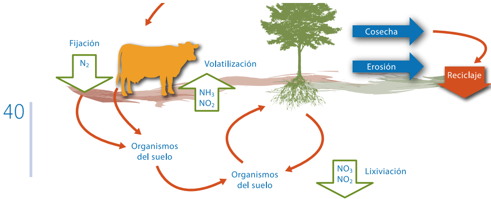
Figura 3.2: Entradas y salidas de Nitrógeno del suelo
