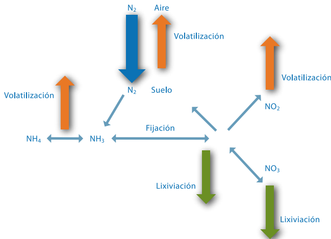
Figura 3.1: Formas de Nitrógeno en el Suelo
