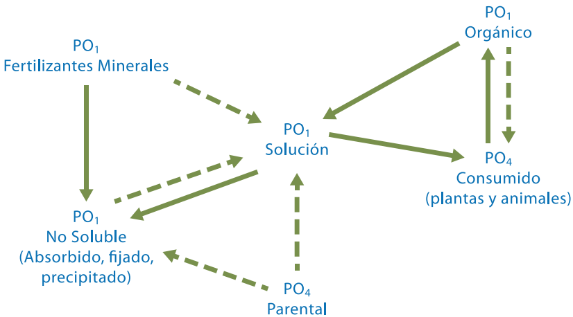
Figura 3.3: Esquema general de las formas de fósforo en el suelo
